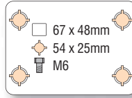
63mm swivel
